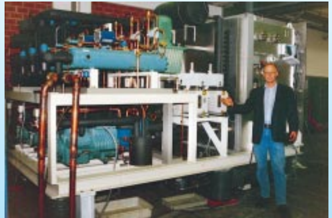
Martin Christ Gefriertrocknungsanlage Typ EPSILON 220 DS
