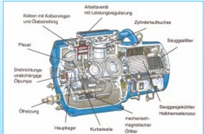
NH 3 -Halbhermetikverdichter von ILKA Mafa
