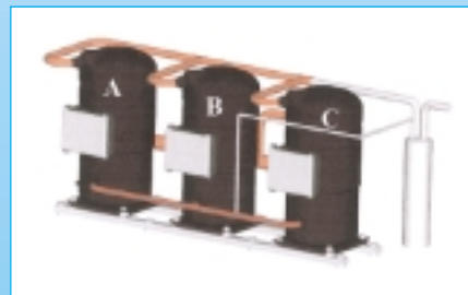
Parallelanwendungen von Scroll-Verdichtern
