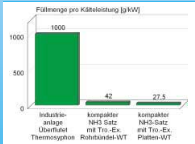
Entwicklung eines NH 3 -Standard-Flüssigkeitskühlsatzes mit minimaler Füllmenge
