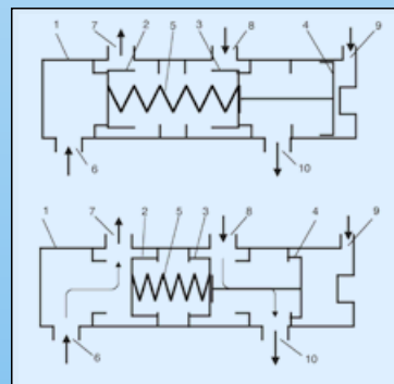
Neues selbsttätiges Absperrventil für Kältemittelverdichter
