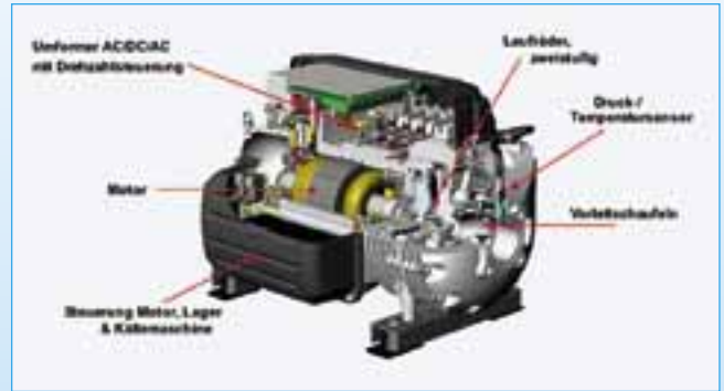
Quantum, eine revolutionäre Turboverdichtertechnologie
