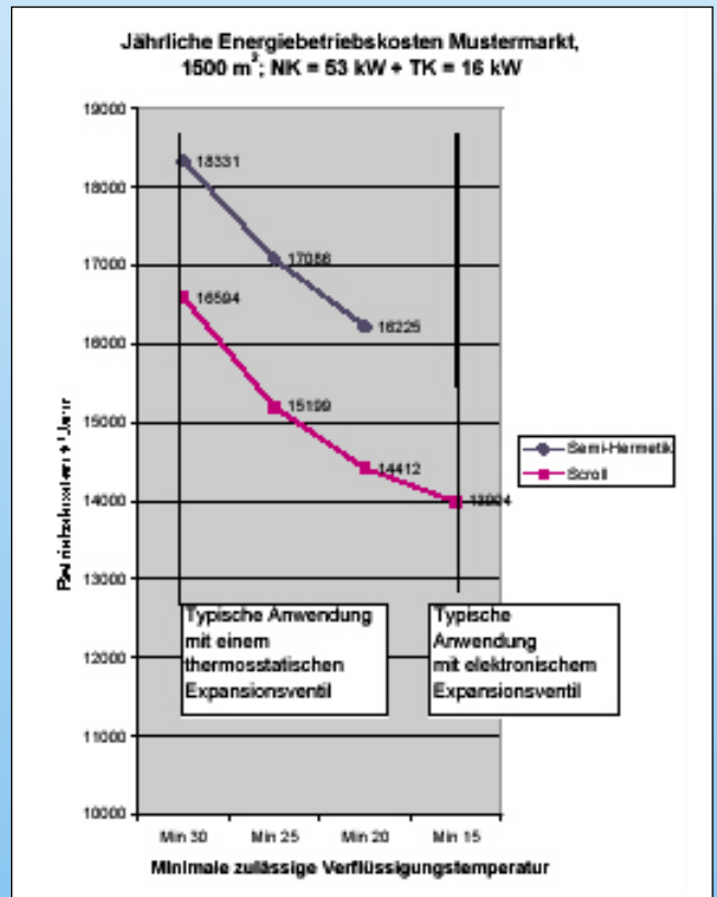
Betrachtung der Investitions- und Energiekosten einer Kälteanlage in einem Supermarkt
