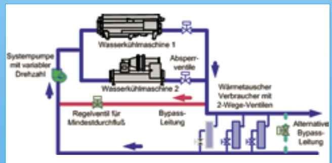
Kaltwasser-Systeme mit variablem Kaltwasser-Volumenstrom
