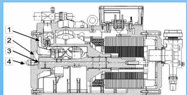
Ein verbessertes Zentrifugal-Schmiersystem für Kältemittelverdichter
