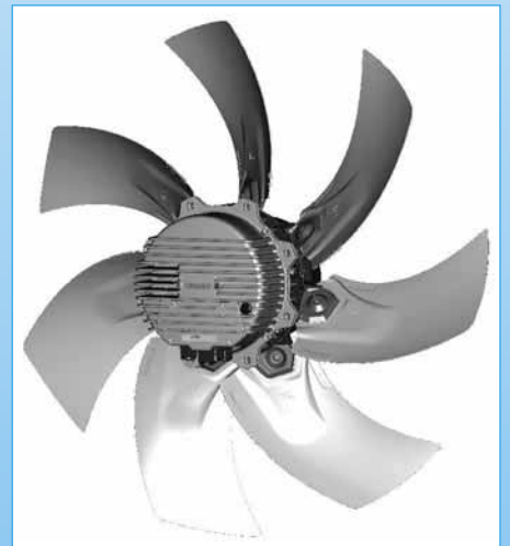
Ventilator: Systemvergleich zwischen Asynchronmotoren und elektronisch kommutierten Motoren
