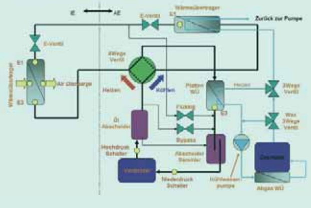
ECO Gas-Wärmepumpe VRF-Multisplit im Holiday Inn Garden Court Helmstedt
