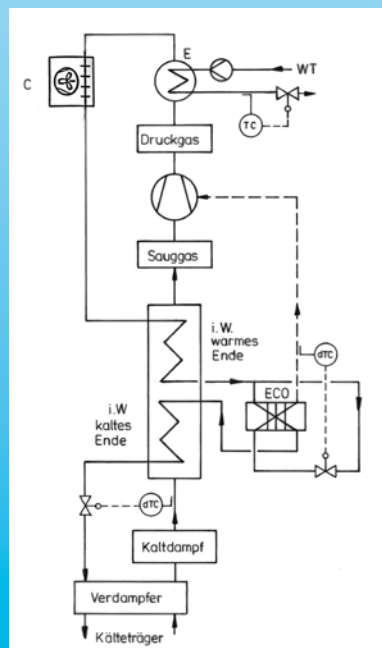
Die wirtschaftliche Kälteanlage
