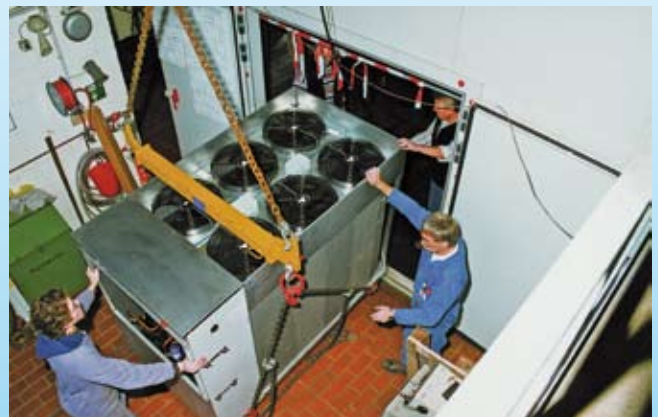
Der kälte- und climatechnische Prüfstand bei DMT
